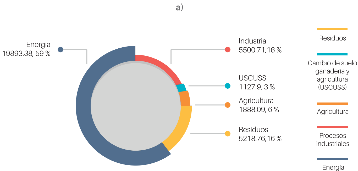
Gráfica 2. Emisiones netas de GEI del estado de Hidalgo por categoría (Ggeq. CO 2 ): a) considera la captura de CO 2 y; b) no considera la captura de CO 2 .
